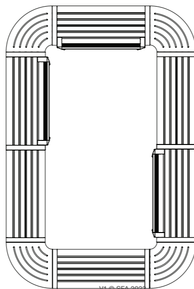
2S-C90-2B-2S-C90-2B-C90-2B-2S-C90
