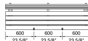
QTY 2
