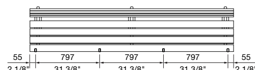
QTY 4
